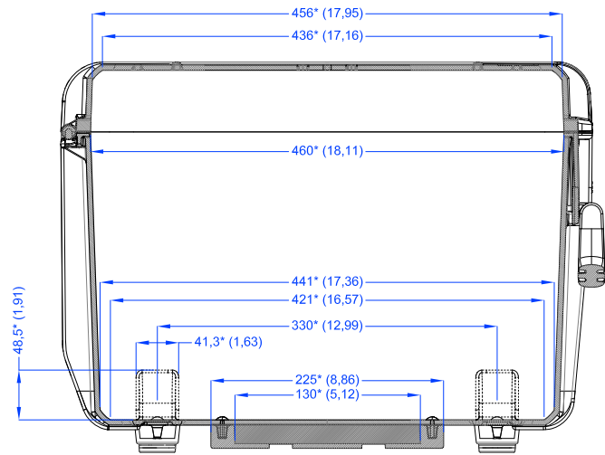
Sezione B-B
