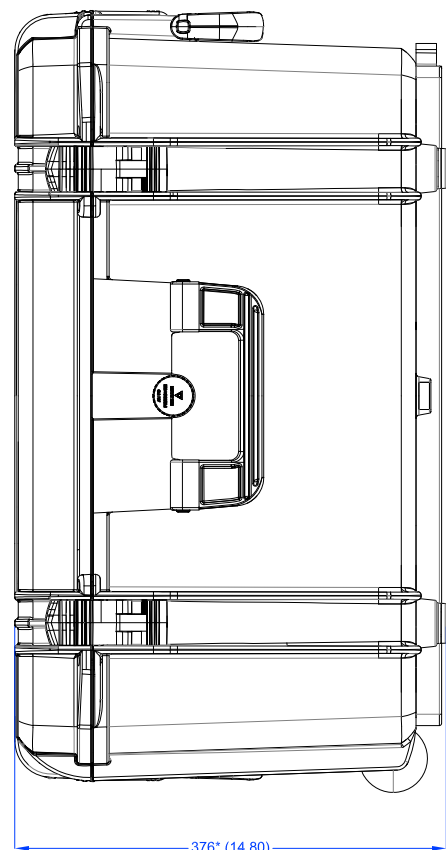
Lato Apertura
