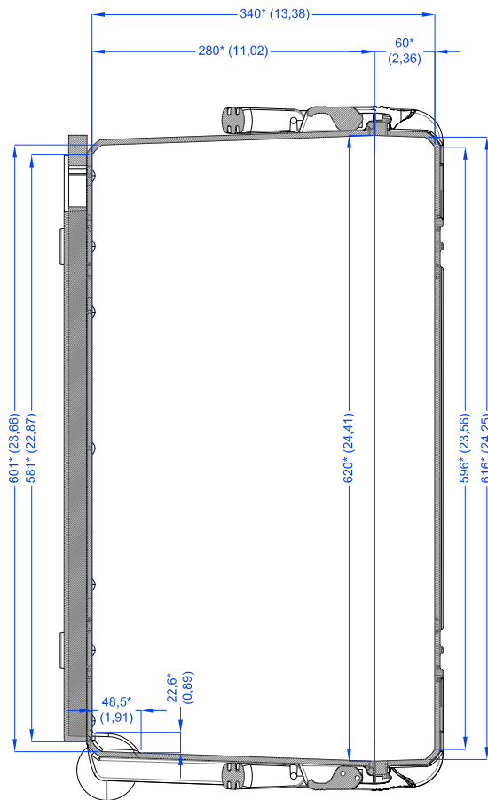
Sezione A-A
