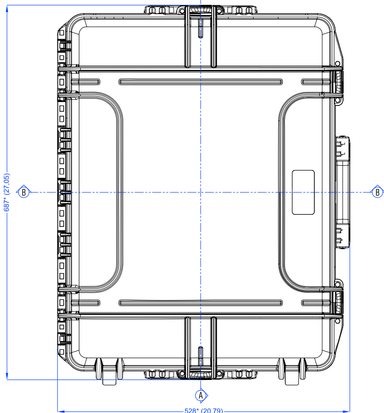
Vista Coperchio
