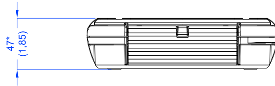
Lato Apertura Opening Side
