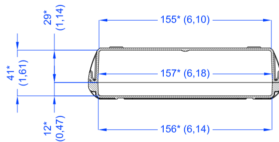
Sezione A-A Section A-A
